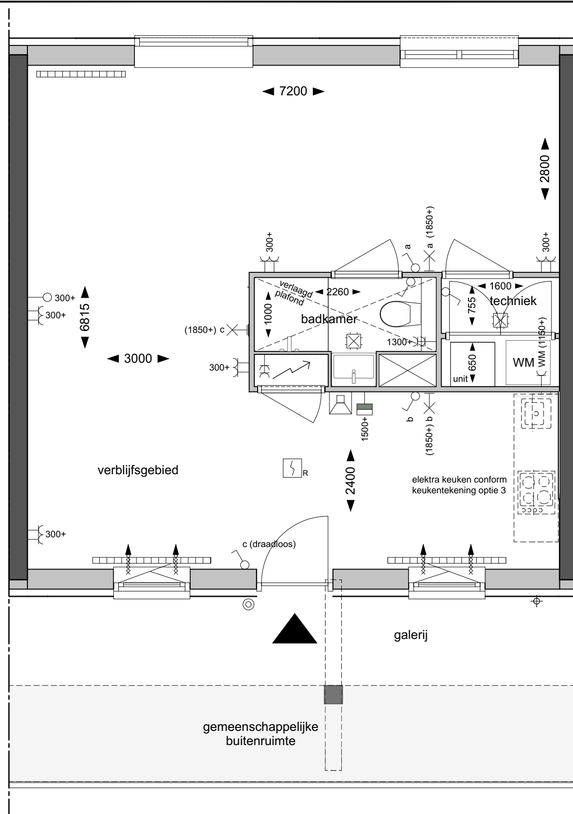
Plattegrond 1:50
