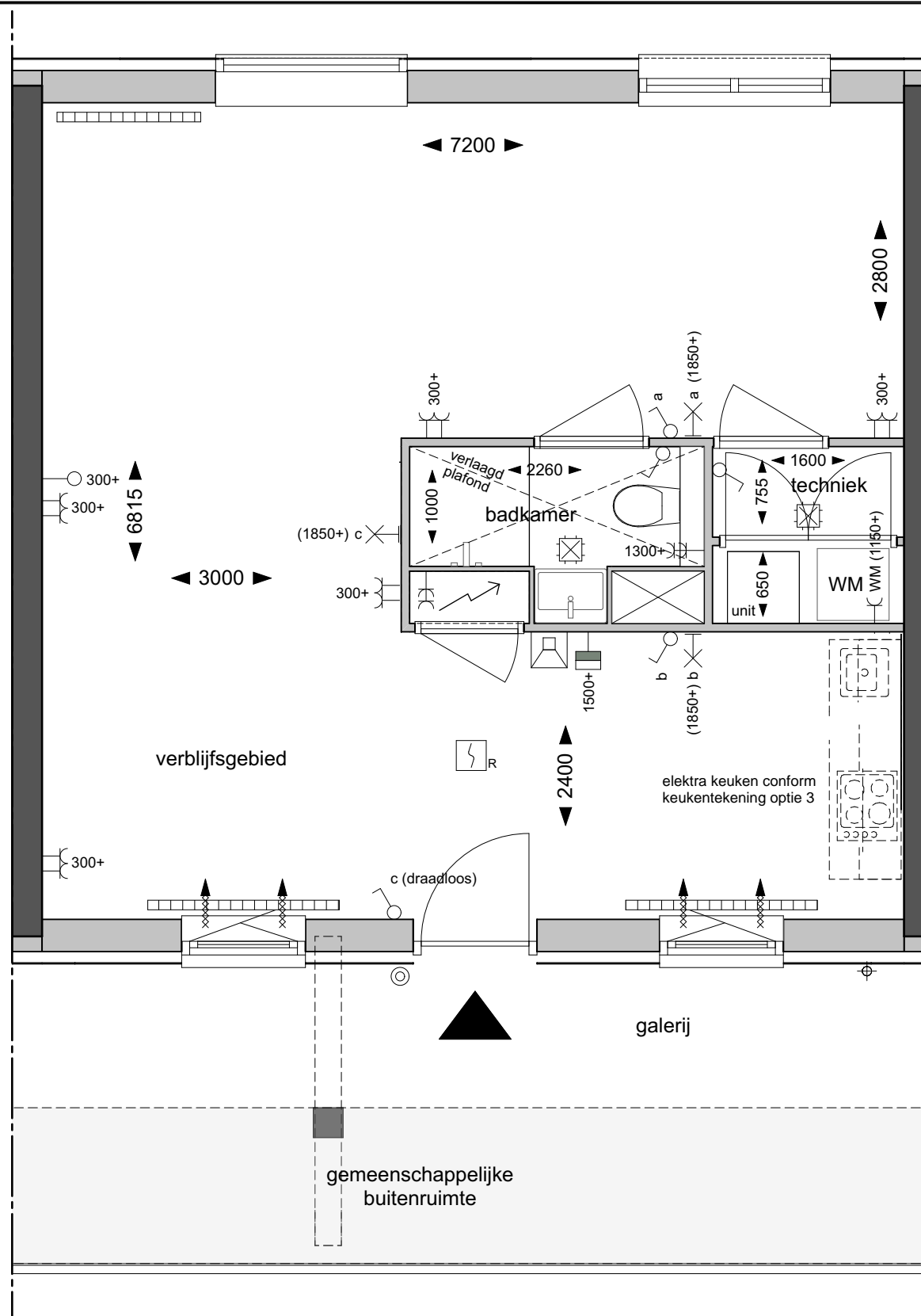
Plattegrond 1:50
