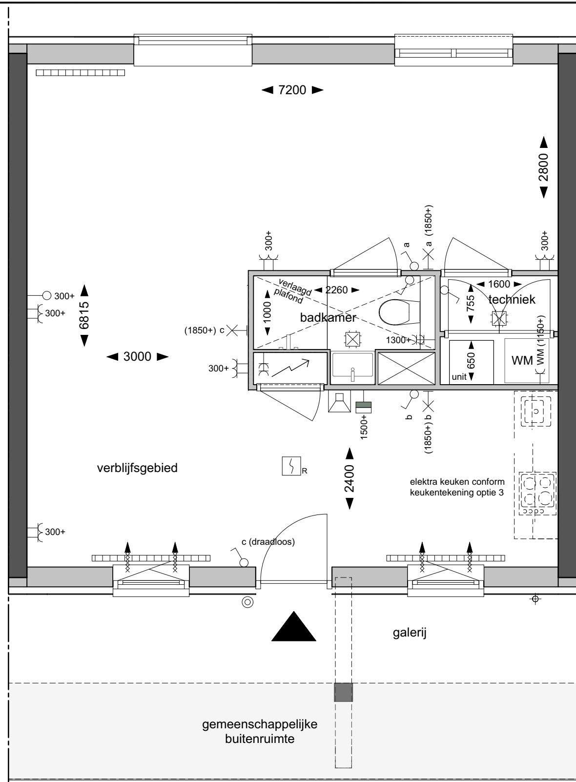
Plattegrond 1:50
