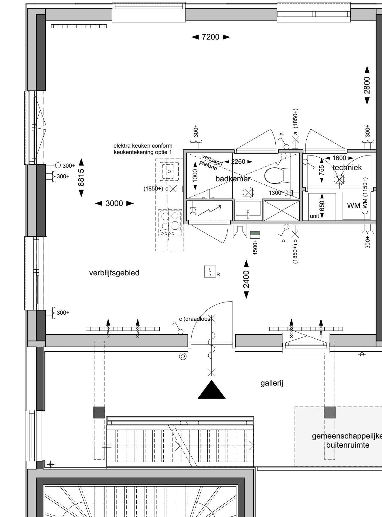
Plattegrond 1:50
