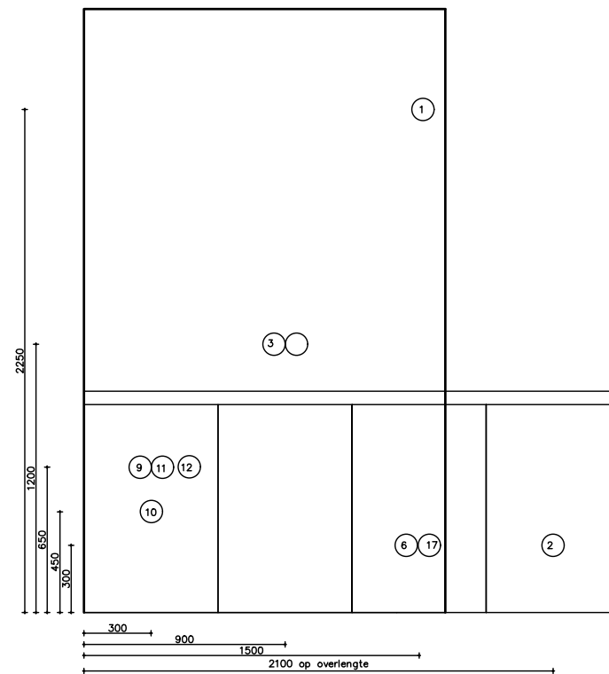
Wandaanzicht
