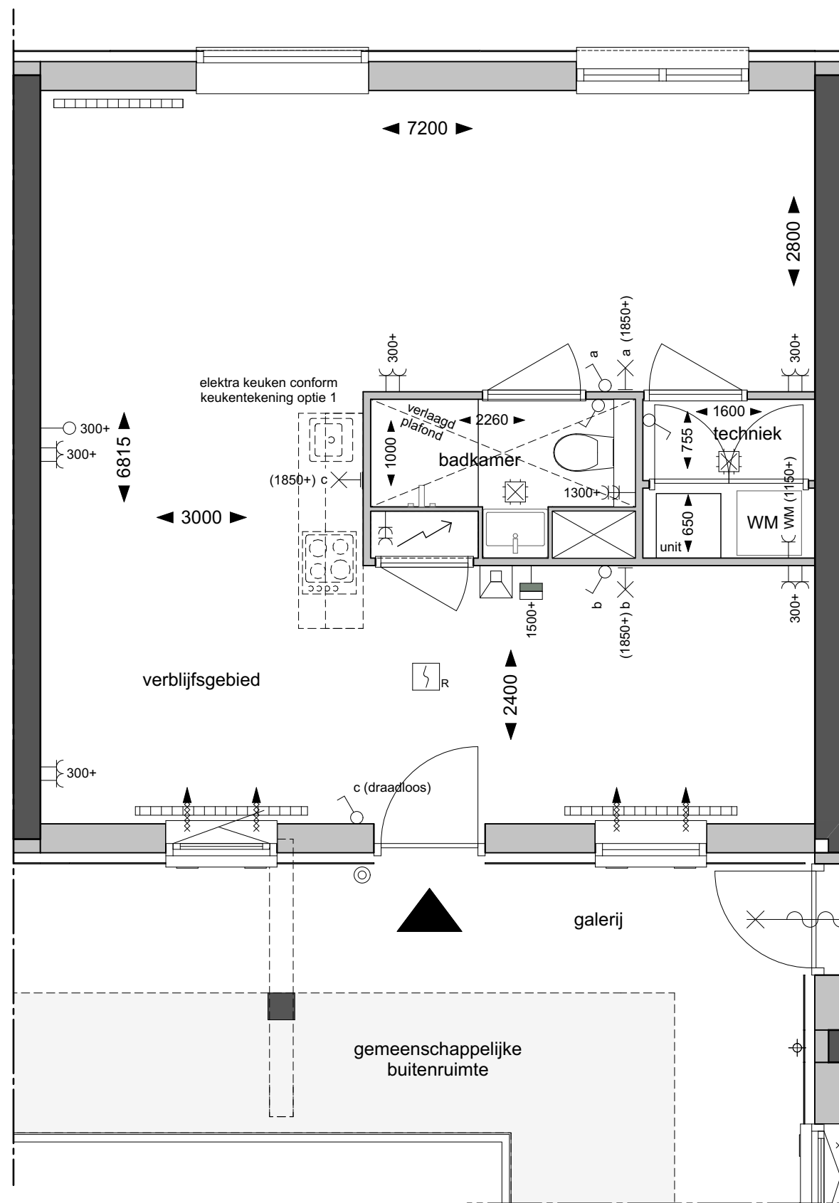
Plattegrond 1:50
