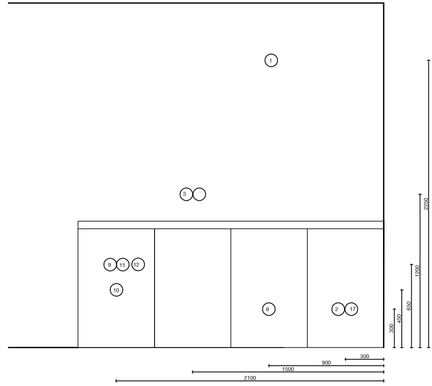
Wandaanzicht
