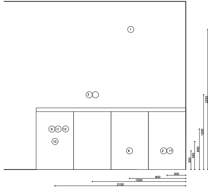
Wandaanzicht
