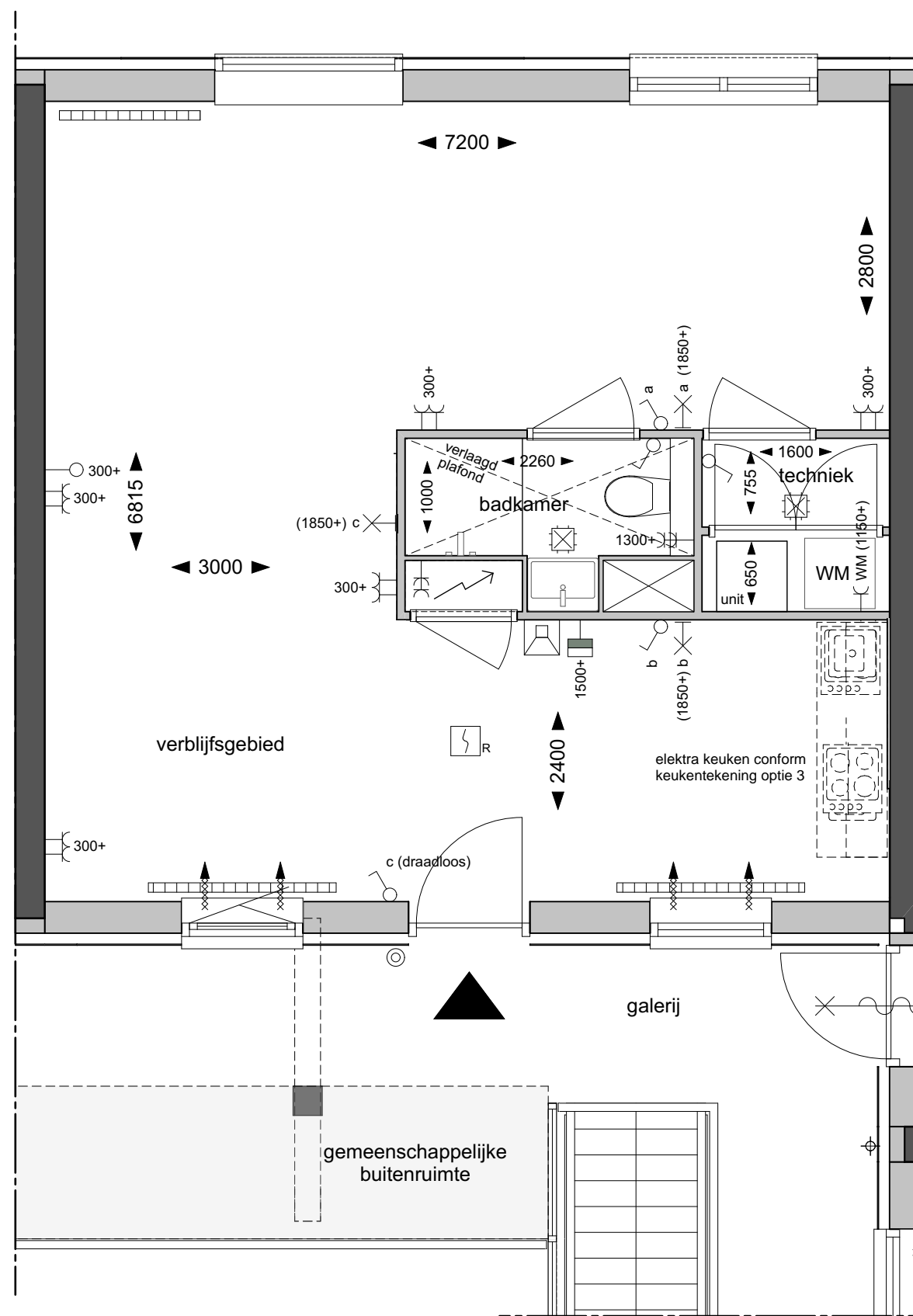
Plattegrond 1:50
